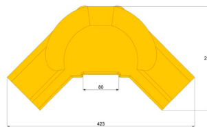
External 90°
